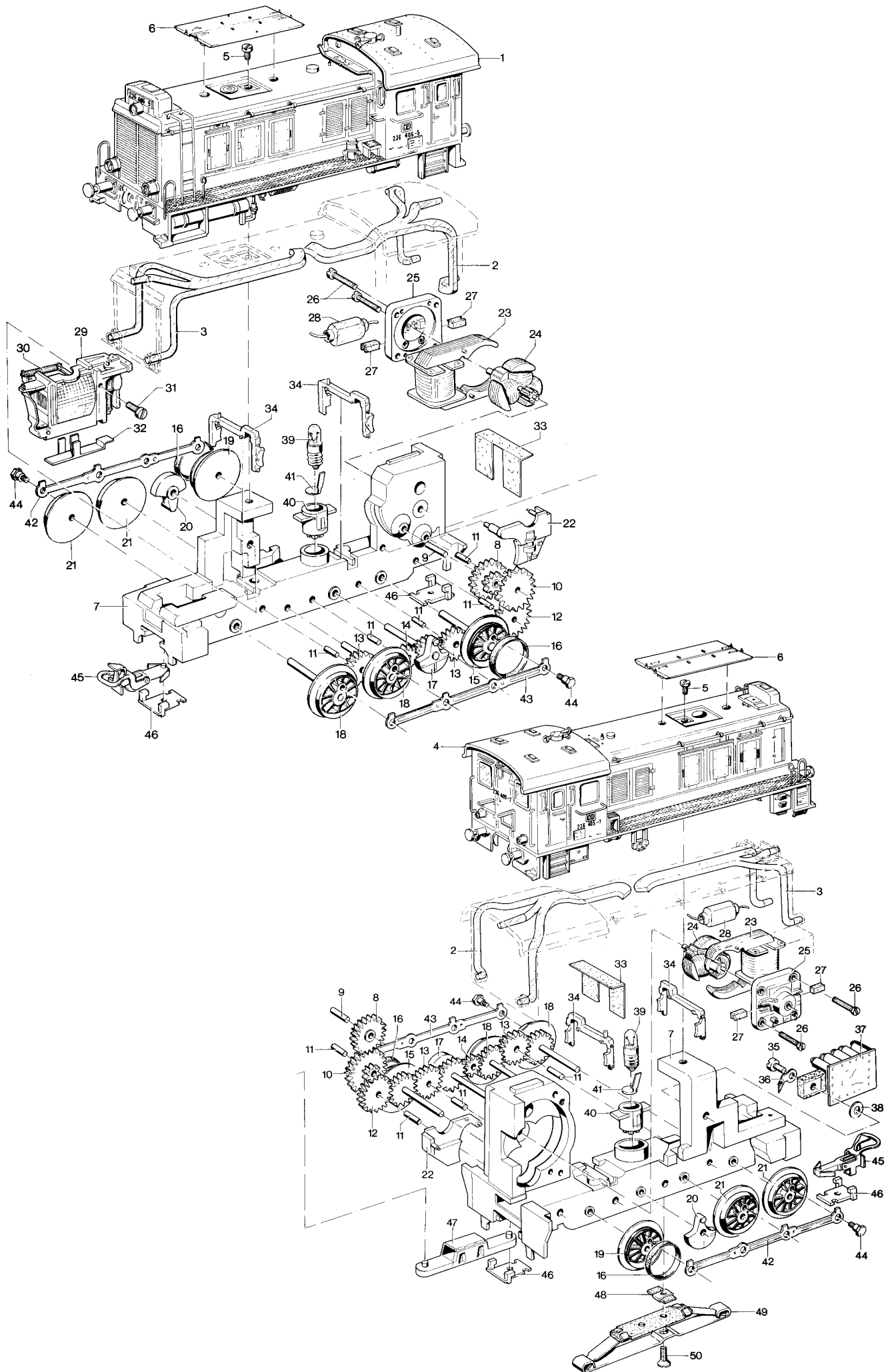
Diesel-Doppellokomotive 3346
